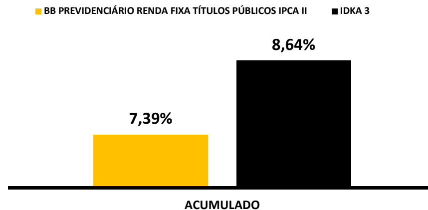
Rentabilidade Acumulada
